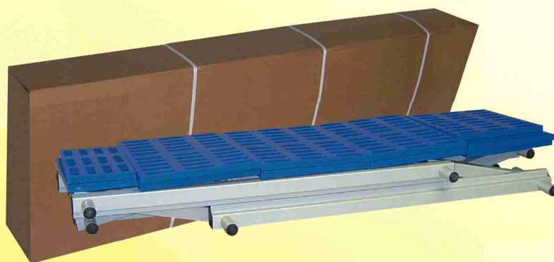
El sistema de plegado permite optimizar el volumen de empaquetado y transporte.
