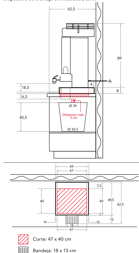
Dispositivo de montaje en mostrador, corte
