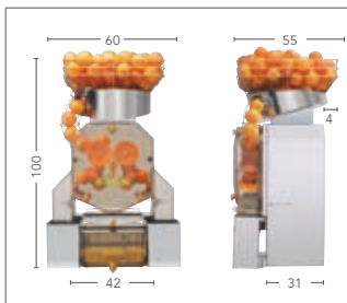
Citrocasa 8000 XB con depósito de zumo N° art. 80.002
